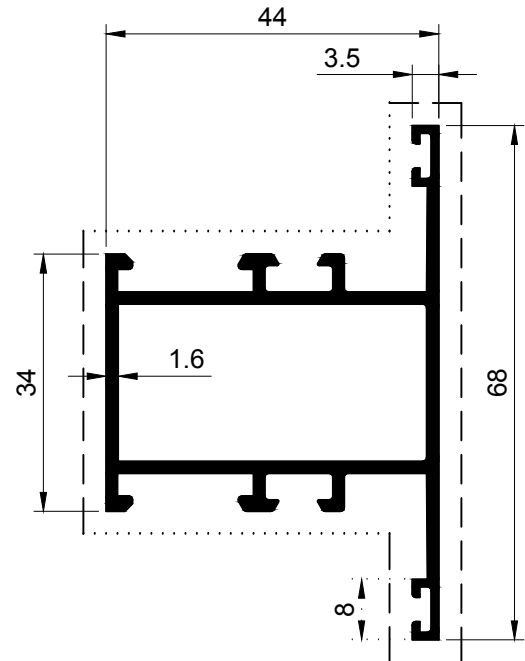
SECTION NO. - ECA-02 EST. WEIGHT - 0.948 KG./M.
