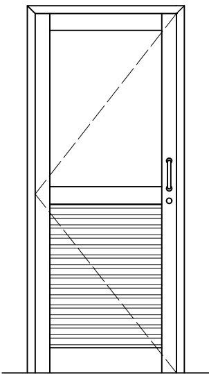
Bottom Louvre
