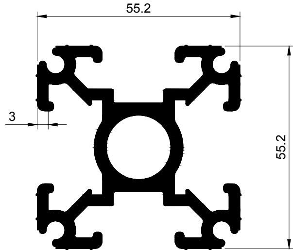
SECTION NO. - HDR-308 EST. WEIGHT - 2.440 KG./M.
