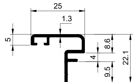
SECTION NO. - SFD-605 EST. WEIGHT - 0.229 KG./M.
