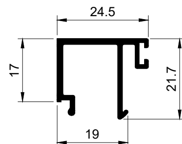
SECTION NO. - GL-124 EST. WEIGHT - 0.285 KG./M. GLASS GAP - 16.0 MM
