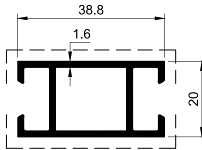
SECTION NO. - ABS-SD06 EST. WEIGHT - 0.550 KG./M.
